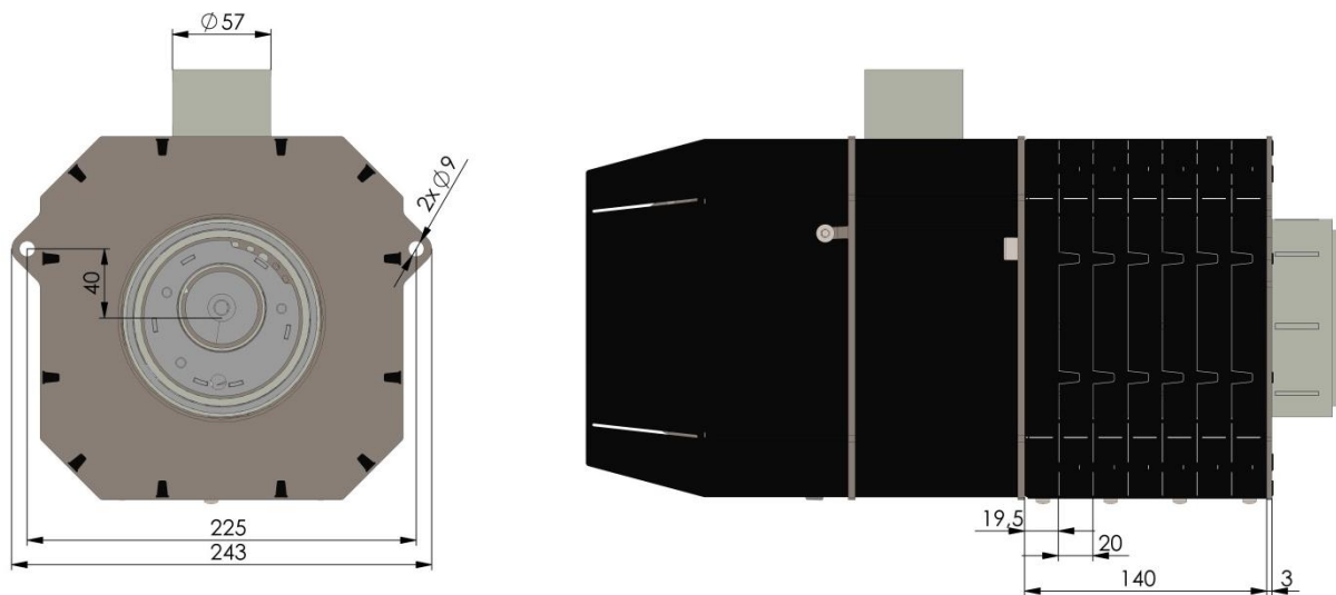
Рис. 21. Вид пальника 20 kW з ізоляційним плащем та монтажною плитою.
