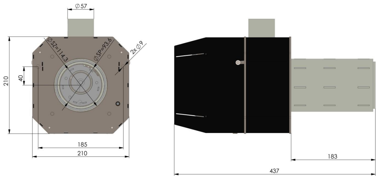
Рис. 20. Вид пальника 20 kW.
