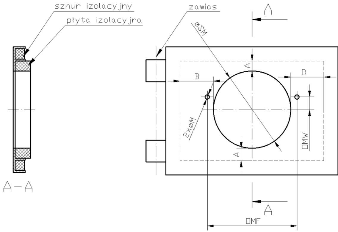
Рис. 4. Схема виконання отворів для пальника з ізоляційним плащем і монтажною плитою для моделей: 16 kW, 20 kW, 26 kW, 36 kW.
