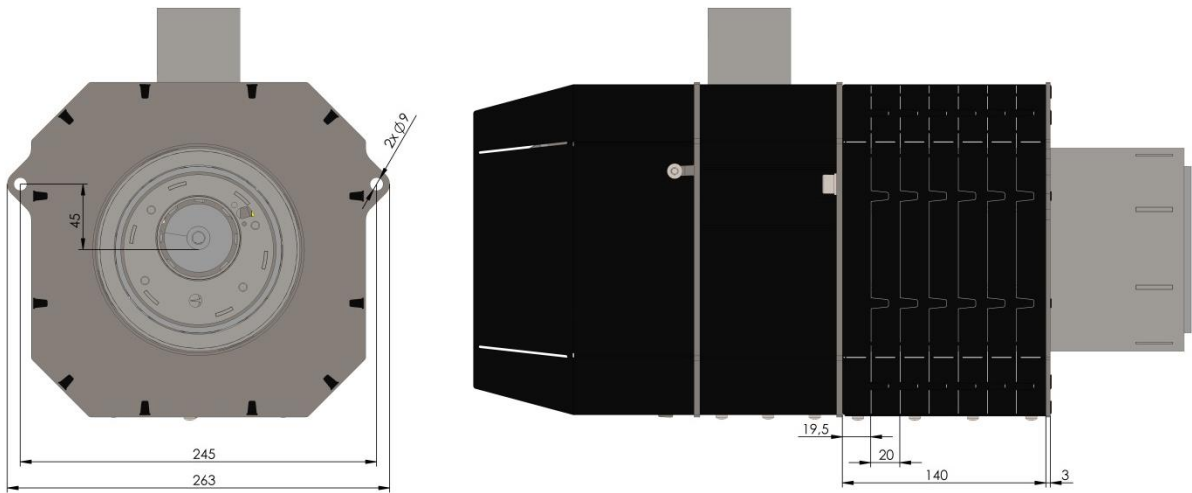
Рис. 24. Вид пальника 36 kW.
