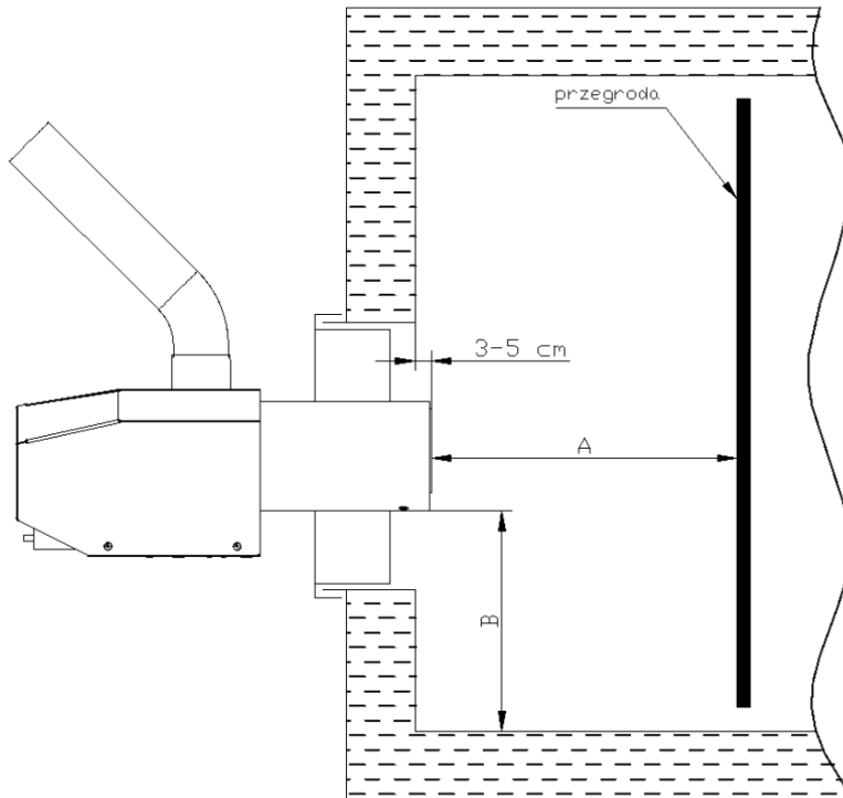
Рис. 7. Вид камери спалювання котла з боку.
