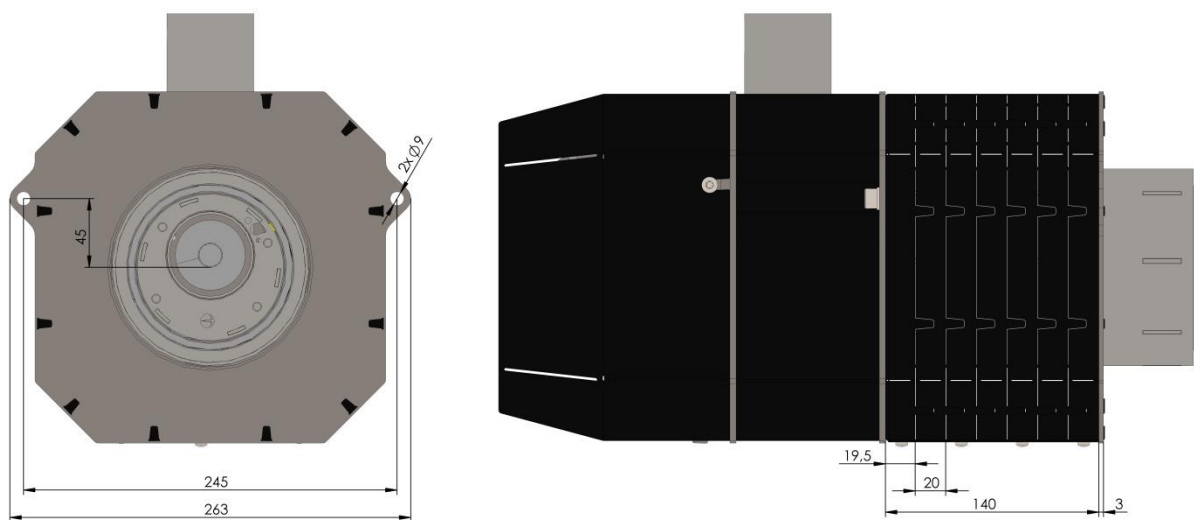
Рис. 23. Вид пальника 26 kW з ізоляційним плащем і монтажною плитою.
