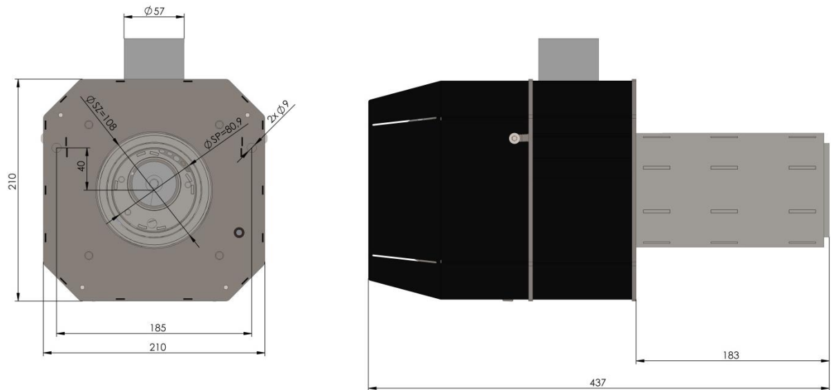
Рис. 18. Вид пальника 16 kW.
