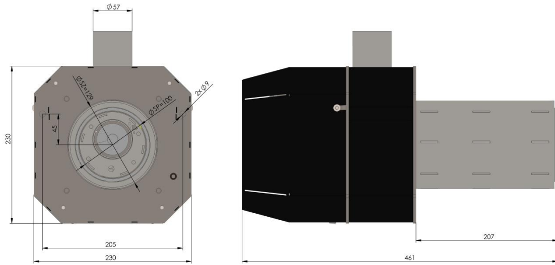
Рис. 22. Вид пальника 26 kW.
