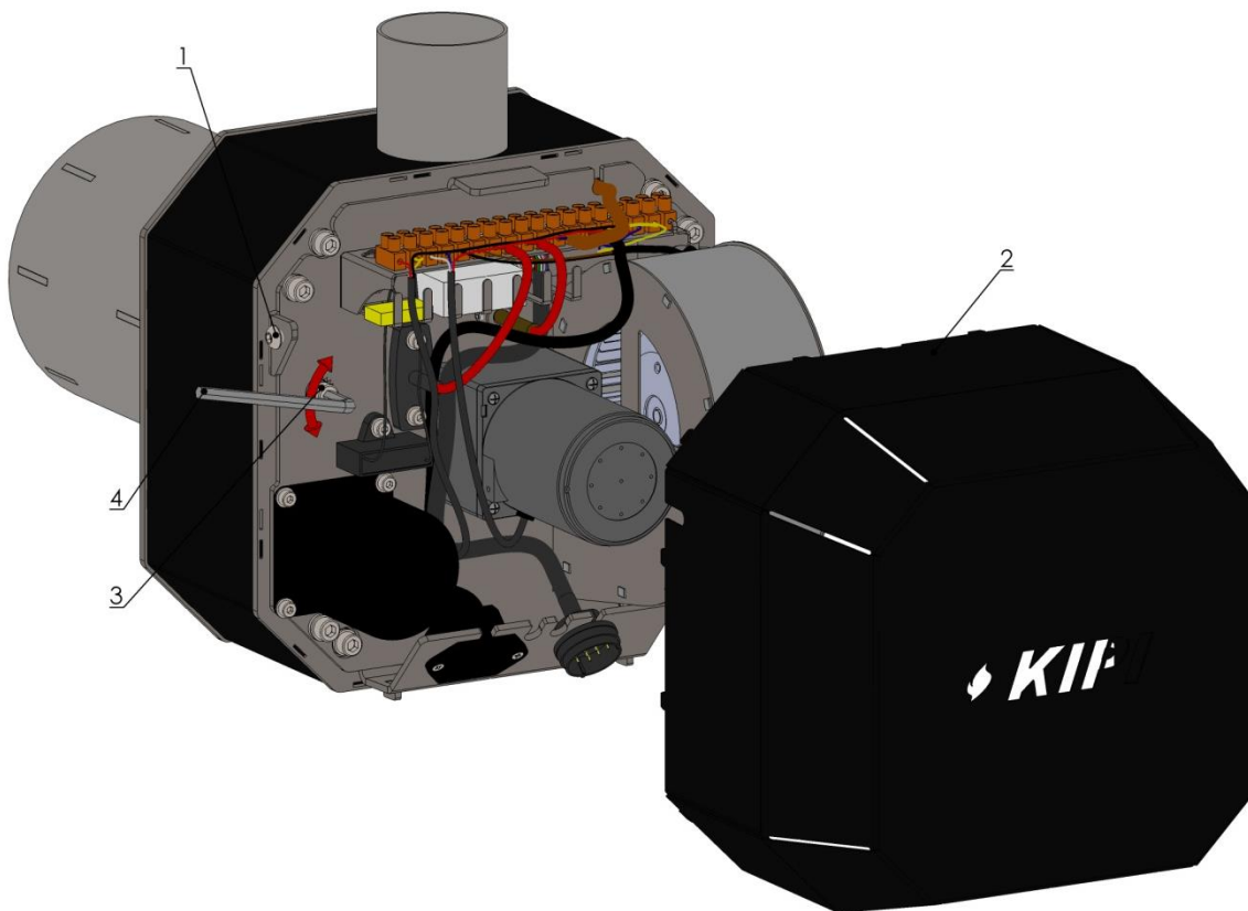
Рис. 10.Регулювання подачі повітря в камеру спалювання.
