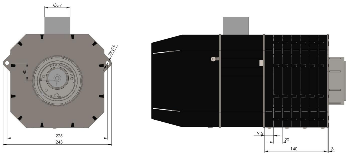
Рис. 19. Вид пальника 16 kW з ізоляційним плащем та монтажною плитою.
