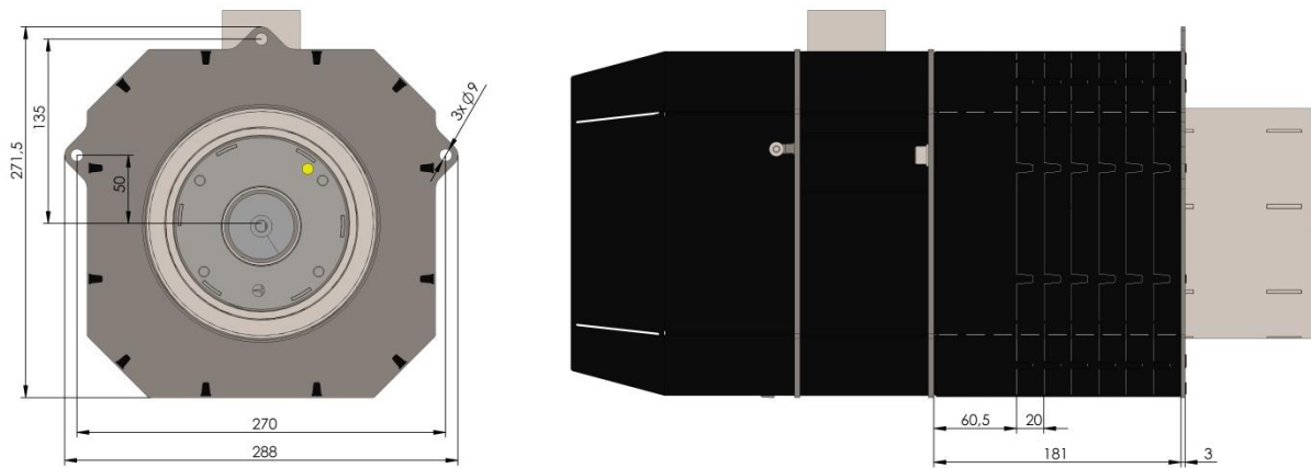
Рис. 27. Вид пальника 50 kW з ізоляційним плащем та монтажною плитою.
